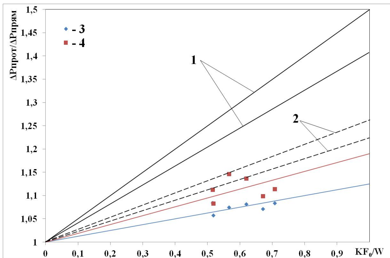
Рисунок 11 – Соотношение потерь давления конденсирующегося пара при прямом и обратном течении: 1 – расчёт по (7), 2 – расчёт по (10), 3 – экспериментальные данные с учётом восстановления давления пара, 4 – экспериментальные данные без учёта восстановления давления пара
