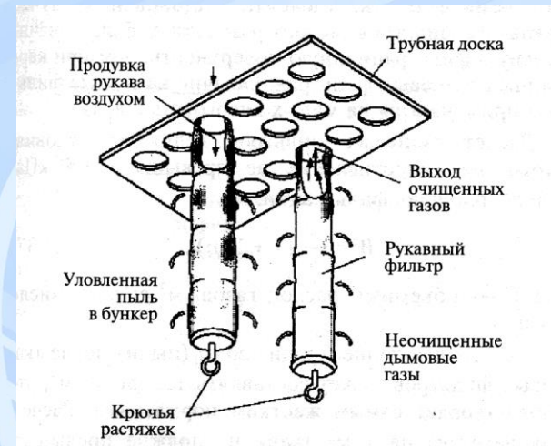
Устройство одной камеры рукавного фильтра.
