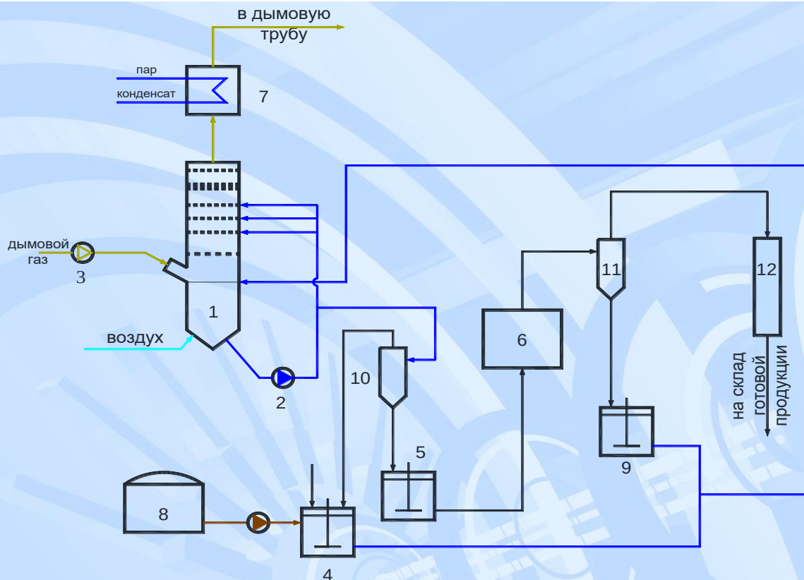
Принципиальная технологическая схема установки аммиачно-сульфатной сероочистки.
